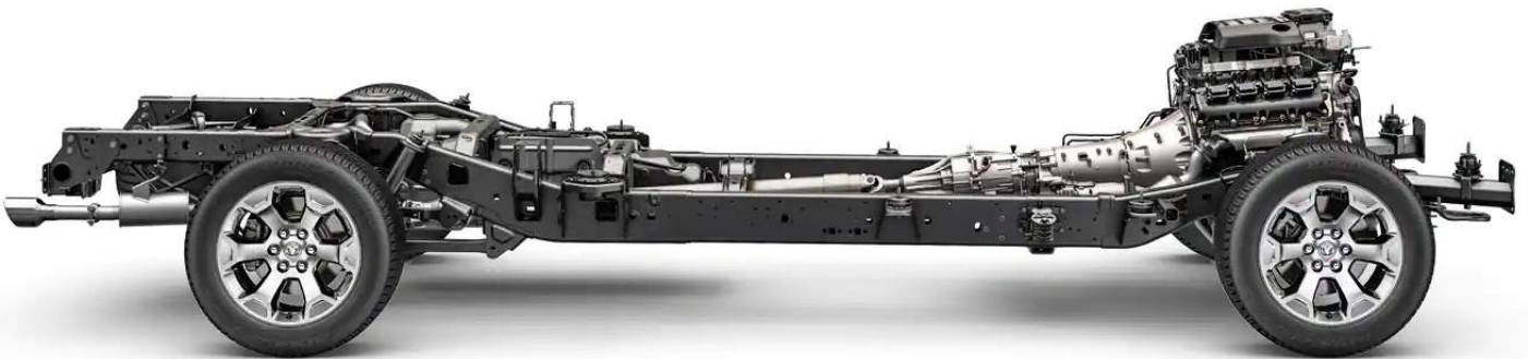
HOGE STERKTE STALEN FRAME DT 2022- Safety-Frame ram 1500
